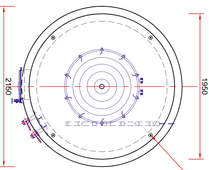
x 4 Douilles d'ancrage
