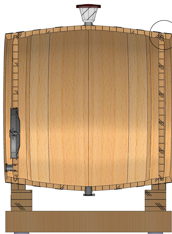
COUPE B-B ECHELLE 1 : 20
