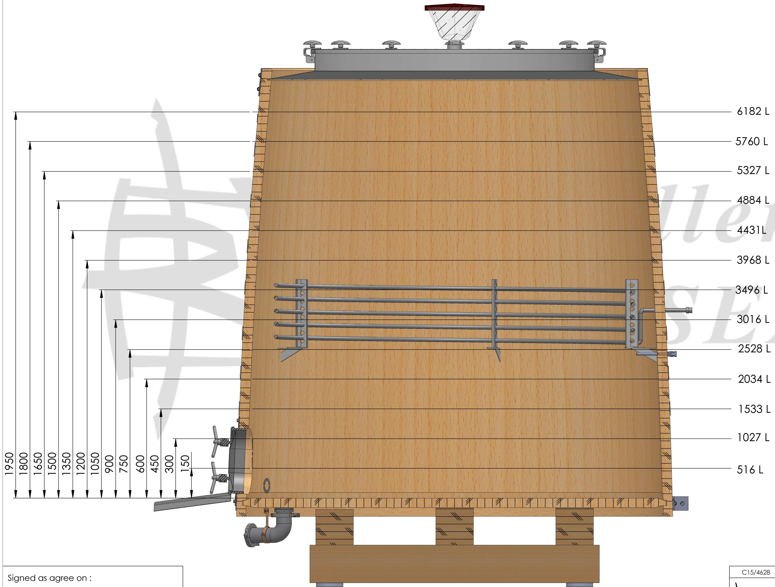
COUPE A-A EHELLE 1 : 12
