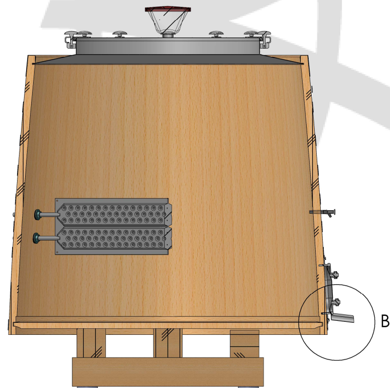
COUPE A-A ECHELLE 1 : 25
