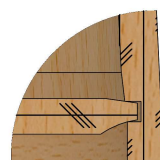
DÉTAIL C ECHELLE 1 : 10
