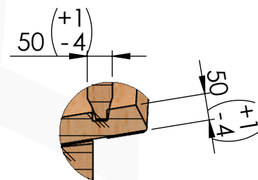
DÉTAIL B ECHELLE 1 : 10
