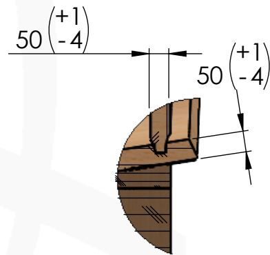
DÉTAIL B ECHÉLLE 2 : 25
