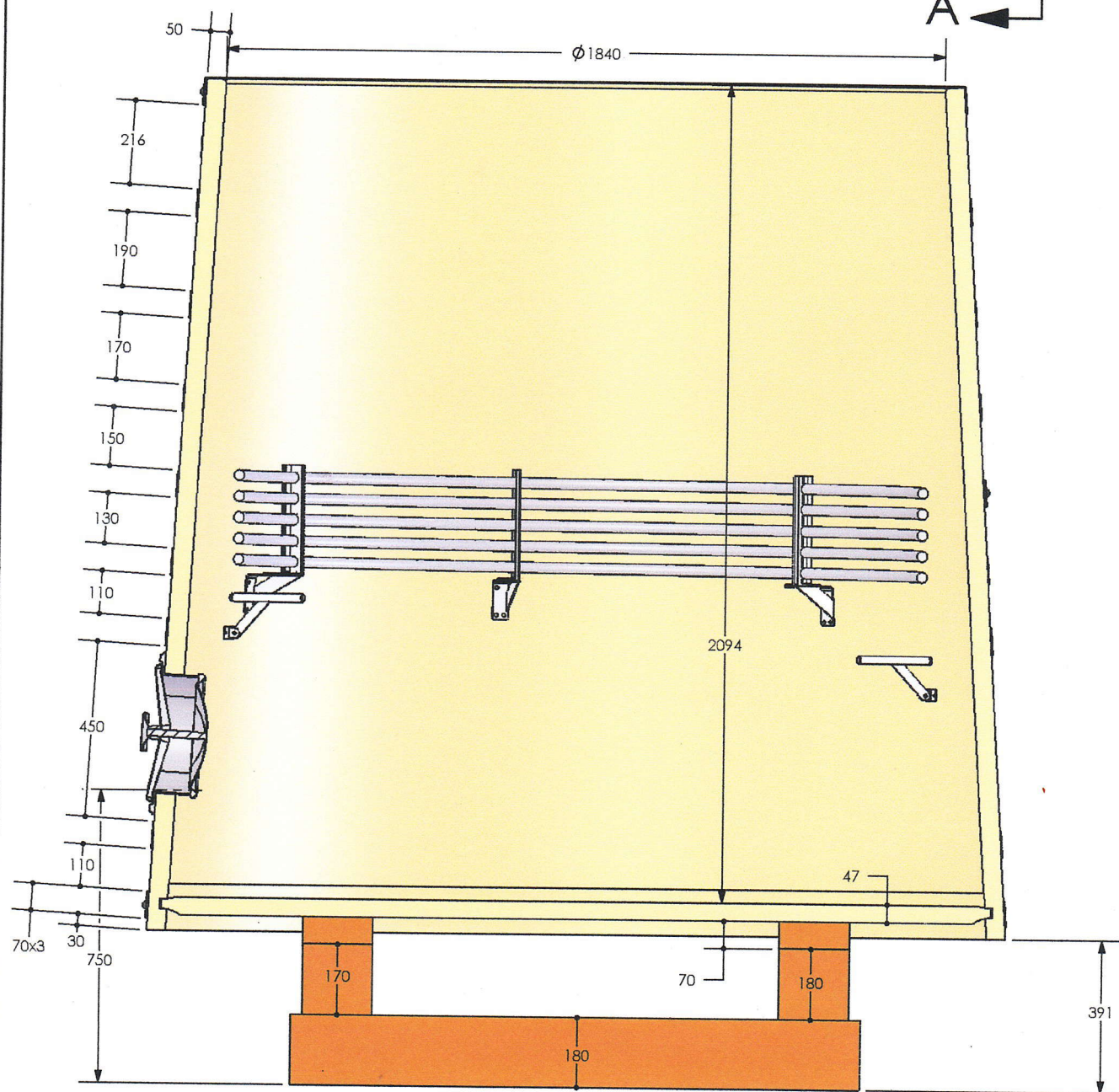
COUPE A-A
